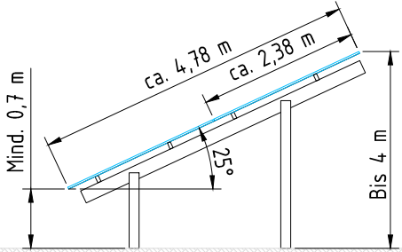
2V - 25° Querschnitt / Cross-section M 1:100
